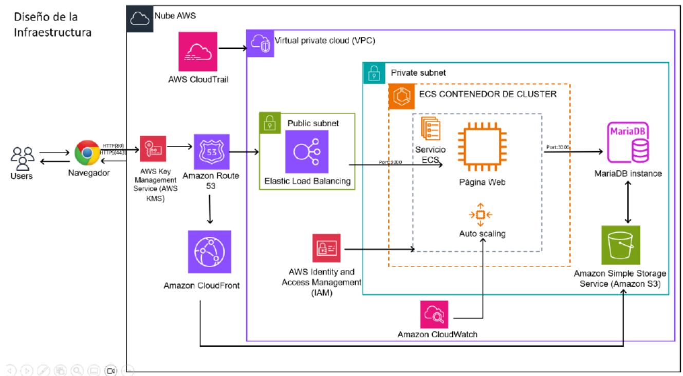
Ejemplo N°4: Diagrama de Arquitectura
